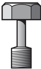
Обработанный болт: когда отверстие с гарантированным зазором слишком мало для регулировки. Part. Nr. D-0002
