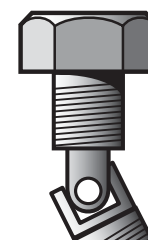
Эластичный болт: растягивается при закручивании Part. Nr. D-0015
