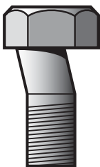
Для отверстий с гарантированным зазором, просверленных наискось Part. Nr. D-0007
